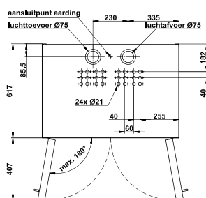
Bovenaanzicht G30.205.090.CLASSIC
