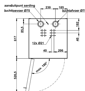
Bovenaanzicht G30.205.060.CLASSIC
