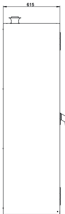
Zijaanzicht G90.205.060.2F.ULTIMATE
