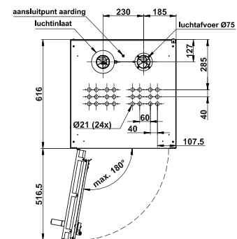
Bovenaanzicht G90.205.060.2F.ULTIMATE
