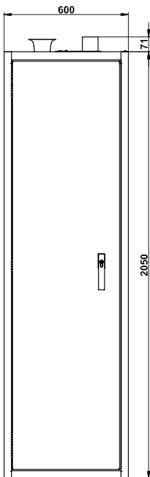
Vooraanzicht G90.205.060.2F.ULTIMATE
