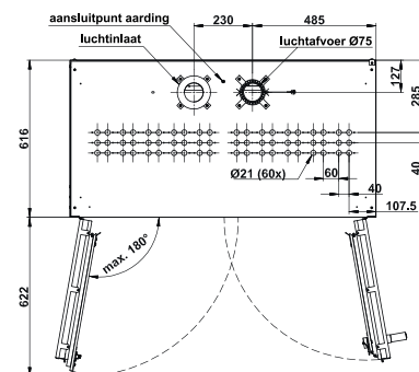
Bovenaanzicht G90.205.120.ULTIMATE
