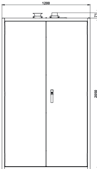
Vooraanzicht G90.205.120.ULTIMATE
