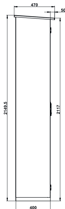
Zijaanzicht G.215.070
