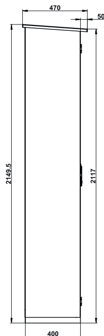
Zijaanzicht G.215.135
