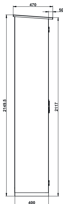
Zijaanzicht G.215.100
