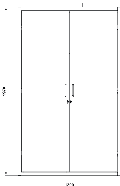
Vooraanzicht SL.196.060.CLASSIC
