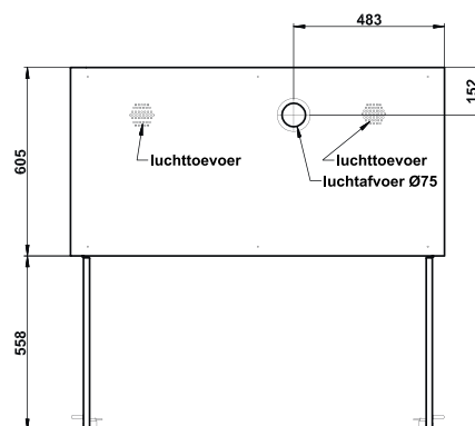
Bovenaanzicht SL.196.120.CLASSIC
