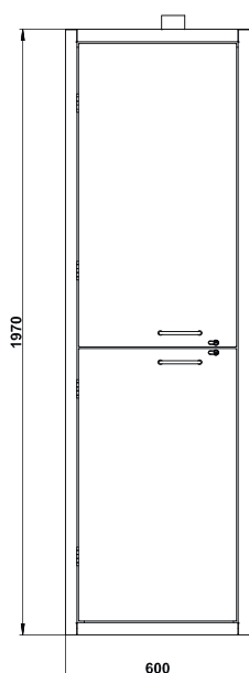
Vooraanzicht SL.196.060.CLASSIC
