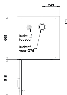
Bovenaanzicht SL.196.060.CLASSIC
