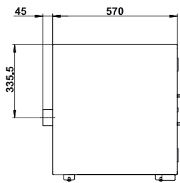
Zijaanzicht SL.060.059.UB.CLASSIC
