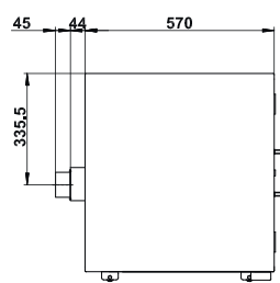
Zijaanzicht SL.060.110.UB.CLASSIC
