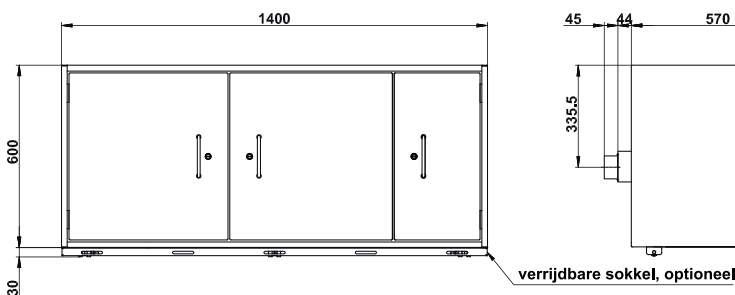
Vooraanzicht SL.060.140.UB.CLASSIC
