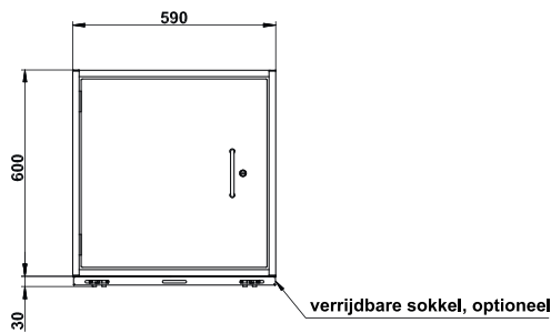
Vooraanzicht SL.060.110.UB.CLASSIC
