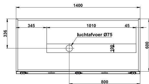
Achteraanzicht SL.060.140.UB.CLASSIC
