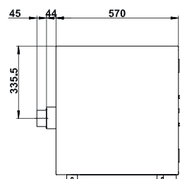
Zijaanzicht SL.060.140.UB.CLASSIC
