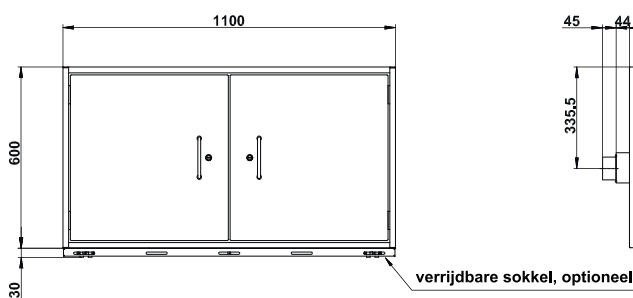
Vooraanzicht SL.060.110.UB.CLASSIC
