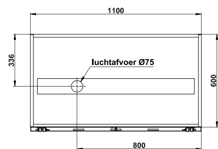
Achteraanzicht SL.060.110.UB.CLASSIC
