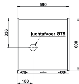
Achteraanzicht SL.060.059.UB.CLASSIC
