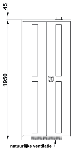
CS.195.081.CLASSIC Vooraanzicht
