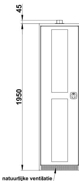
CS.195.054.A.CLASSIC Vooraanzicht
