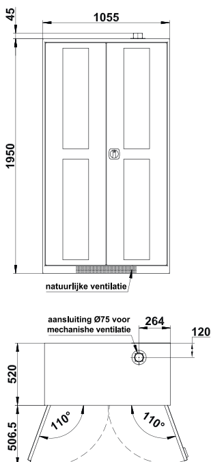
CS.195.105.A.CLASSIC Vooraanzicht / bovenaanzicht
