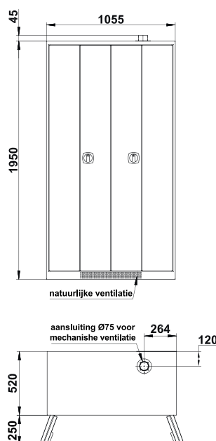
CS.195.105.CLASSIC Vooraanzicht / bovenaanzicht
