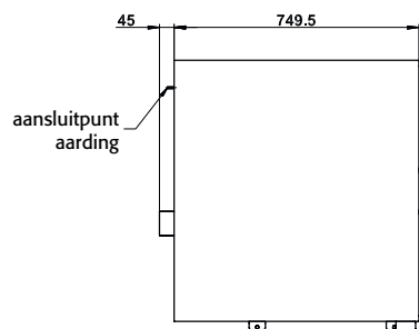
Zijaanzicht UB90.080.110.075.2T
