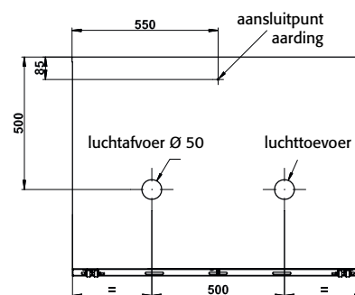
Achteraanzicht UB90.080.110.075.2T
