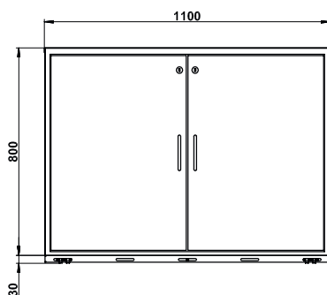
Vooraanzicht UB90.080.110.075.2T
