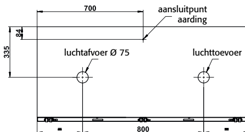
Achteraanzicht UB30.060.110.2T
