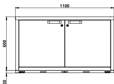
Vooraanzicht UB30.060.110.2T
