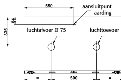
Achteraanzicht UB30.060.110.2T
