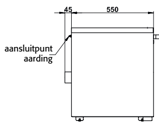
Zijaanzicht UB30.060.110.2T
