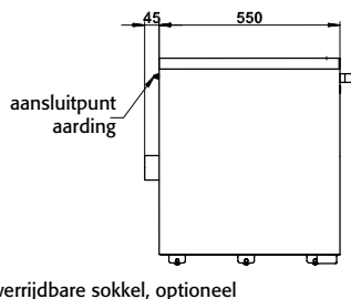
Zijaanzicht UB30.060.110.2T
