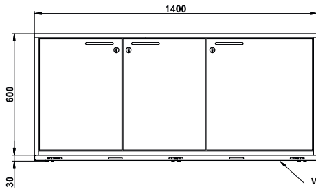
Vooraanzicht UB90.060.140.S2T
