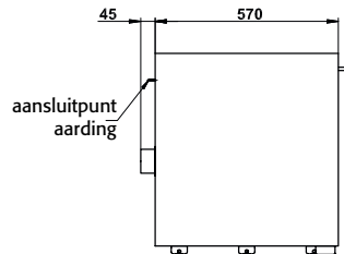
Zijaanzicht UB90.060.140.S2T
