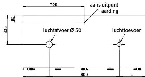
Achteraanzicht UB90.060.140.050.S2T
