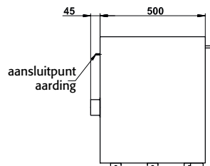
Zijaanzicht UB90.060.140.050.S2T
