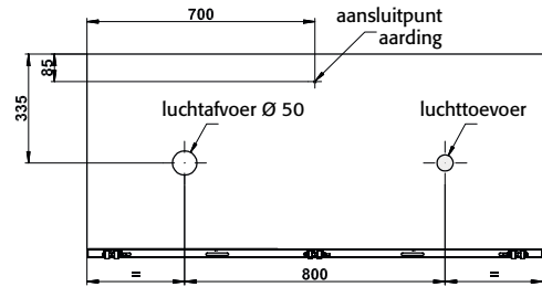
Achteraanzicht UB90.060.140.S2T
