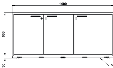
Vooraanzicht UB90.060.140.050.S2T
