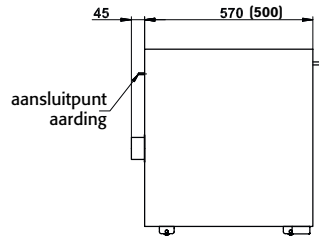
Zijaanzicht UB90.060.059(.050).S
