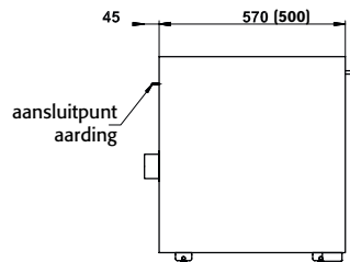
Zijaanzicht UB90.060.059(.050).T
