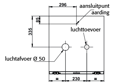
Achteraanzicht UB90.060.059(.050).T
