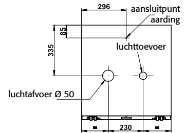
Achteraanzicht UB90.060.059(.050).T
