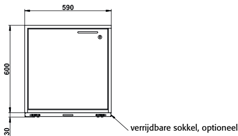
Vooraanzicht UB90.060.059(.050).T
