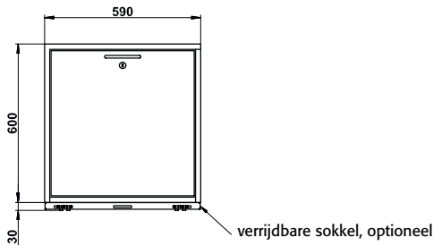
Vooraanzicht UB90.060.059(.050).T
