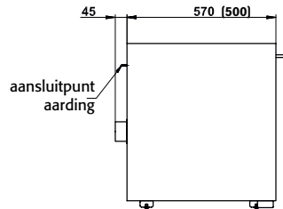
Zijaanzicht UB90.060.110(.050).S
