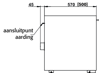
Zijaanzicht UB90.060.110(.050).2S
