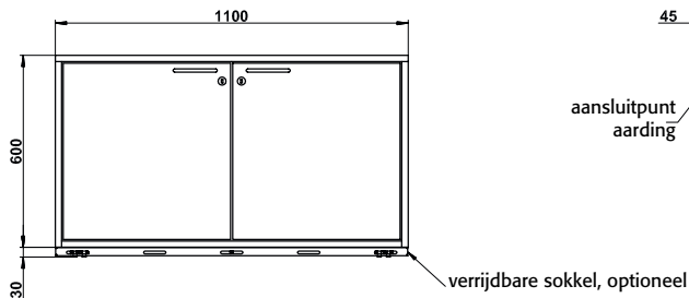
Vooraanzicht UB90.060.110(.050).2S
