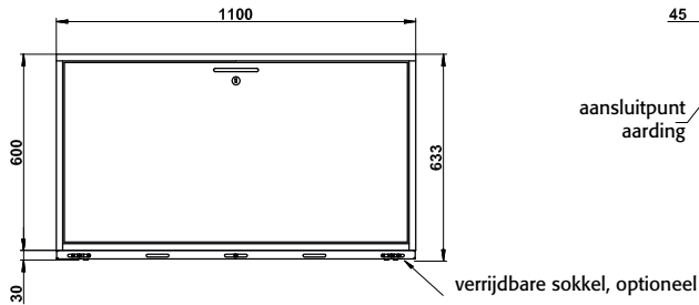
Vooraanzicht UB90.060.110(.050).2S
