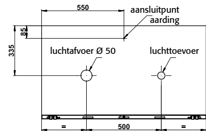
Achteraanzicht UB90.060.110(.050).2S
