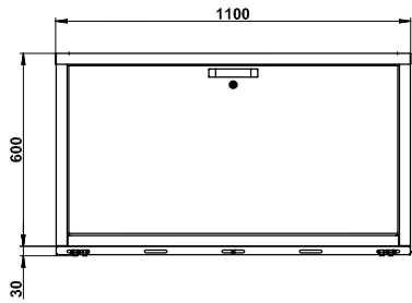
Vooraanzicht UB30.060.110.S
