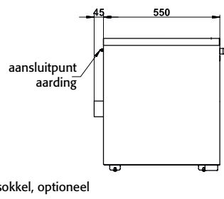
Zijaanzicht UB30.060.110.2S
