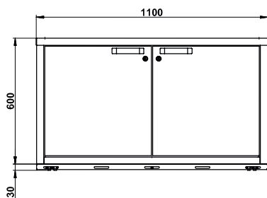
Vooraanzicht UB30.060.110.2S
