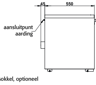
Zijaanzicht UB30.060.110.S
