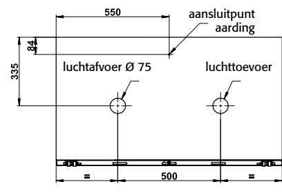
Achteraanzicht UB30.060.110.2S
