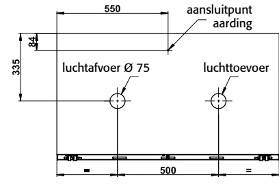
Achteraanzicht UB30.060.110.S
