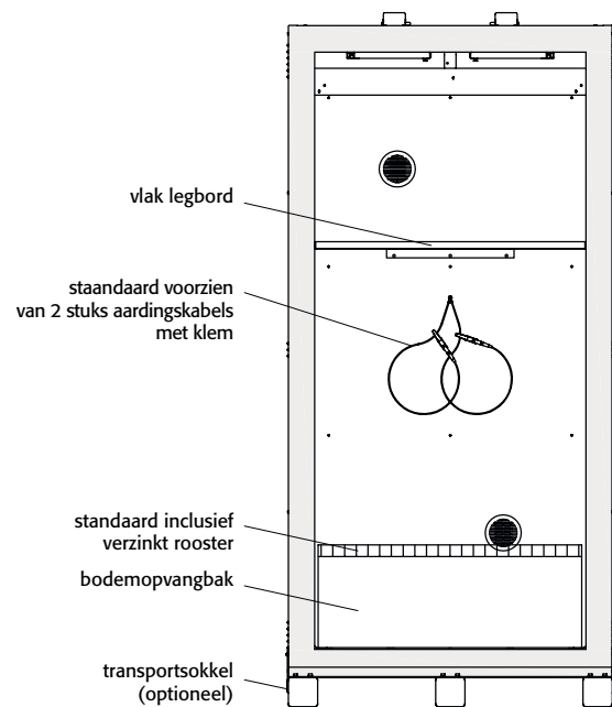
Doorsnede XL90.222.110.CLASSIC
