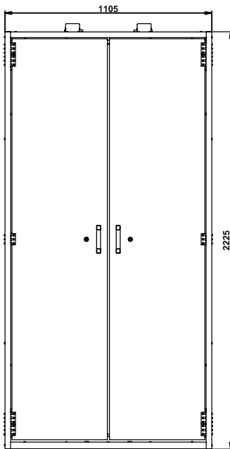
Vooraanzicht XL90.222.110.CLASSIC
