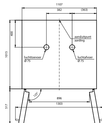
Bovenaanzicht XL90.222.110.CLASSIC
