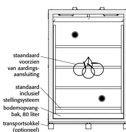
Doorsnede XL90.222.155. CLASSIC met stellingsysteem
