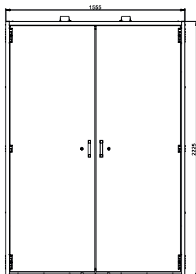
Voor- / zij aanzicht XL90.222.155. CLASSIC
