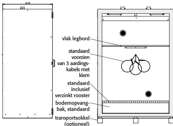
Doorsnede XL90.222.155. CLASSIC met standaard bodempvangbak
