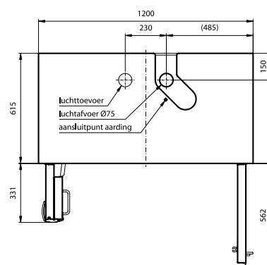
Bovenaanzicht K90.196.120.PHOENIX Vol. 2
