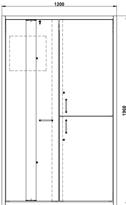
Vooraanzicht K90.196.120.PHOENIX
