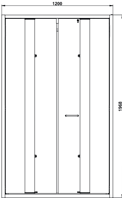
Vooraanzicht S90.196.120.PHOENIX Vol. 2
