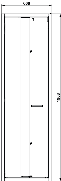
Vooraanzicht S90.196.060.PHOENIX
