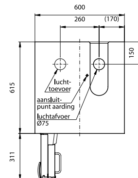
Bovenaanzicht S90.196.060.PHOENIX
