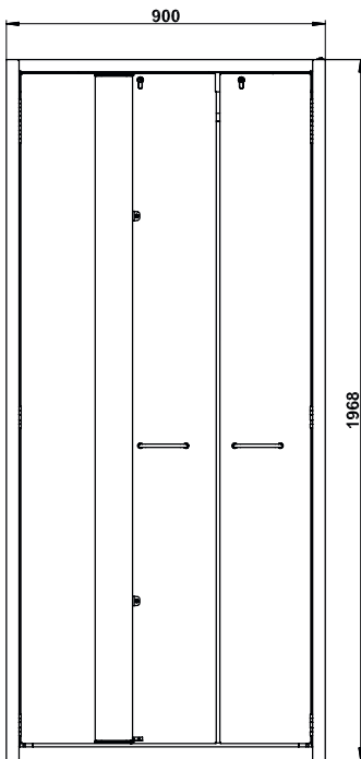
Vooraanzicht S90.196.090.PHOENIX
