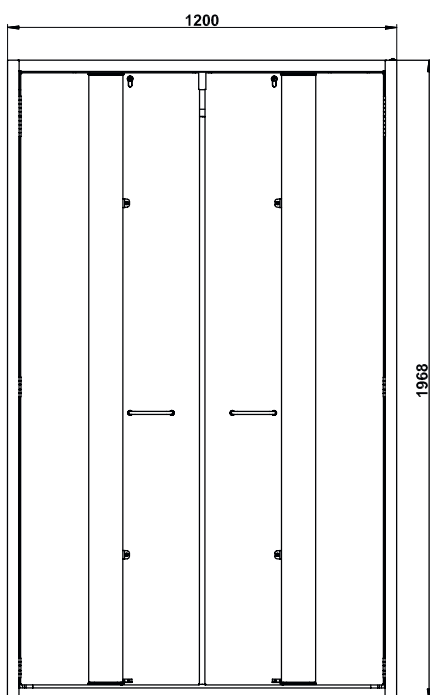
Vooraanzicht S90.196.120.PHOENIX
