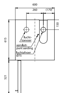
Bovenaanzicht S90.129.060.CLASSIC
