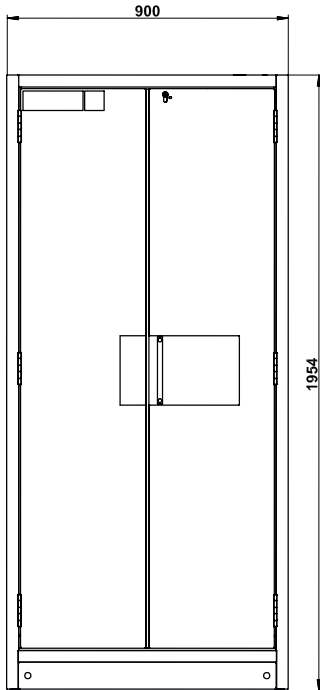
Vooraanzicht Q90.195.090.PEGASUS
