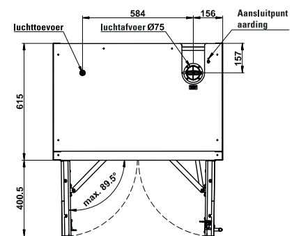
Bovenaanzicht Q90.195.090.PEGASUS
