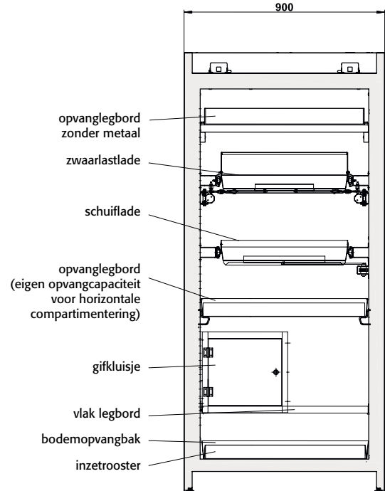
Doorsnede Q90.195.090.PEGASUS
