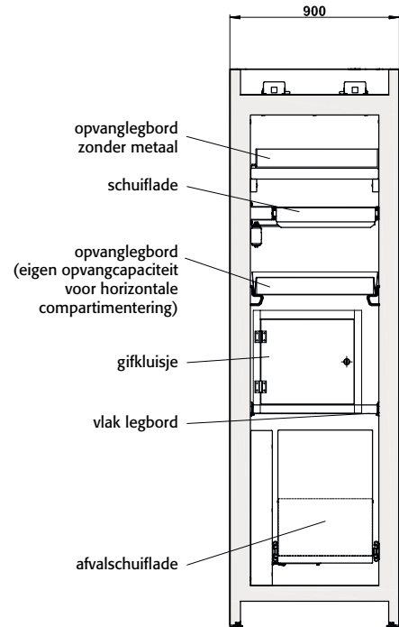
Doorsnede Q90.195.060.PEGASUS
