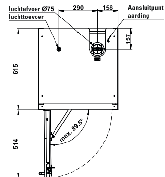
Bovenaanzicht Q90.195.060.PEGASUS
