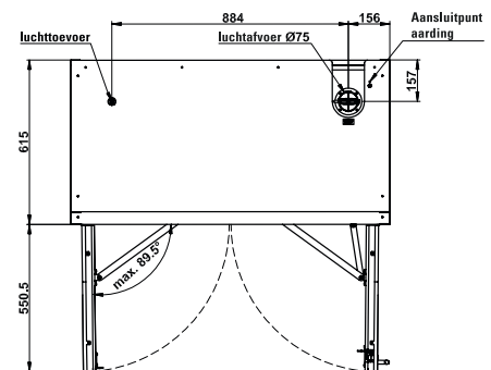
Bovenaanzicht Q90.195.120.PEGASUS
