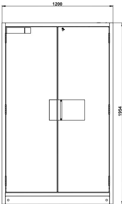
Vooraanzicht Q90.195.120.PEGASUS
