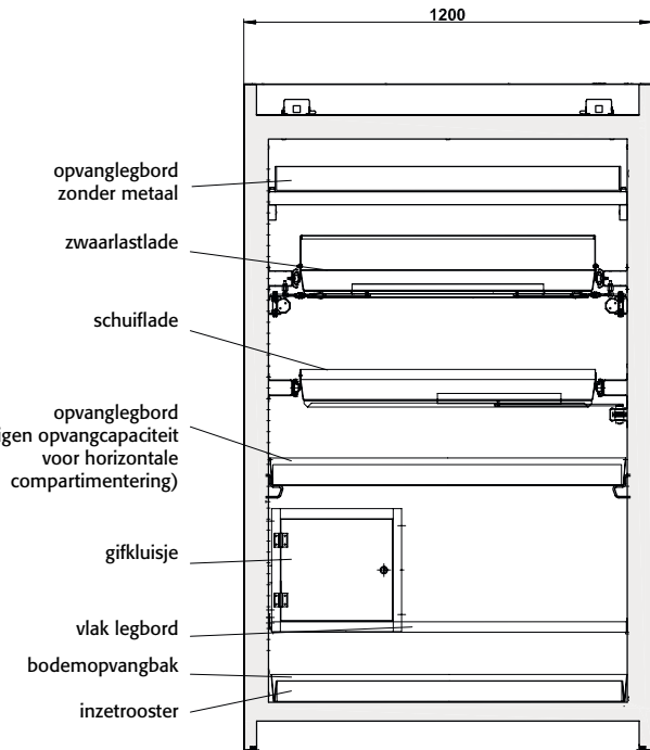
Doorsnede Q90.195.120.PEGASUS
