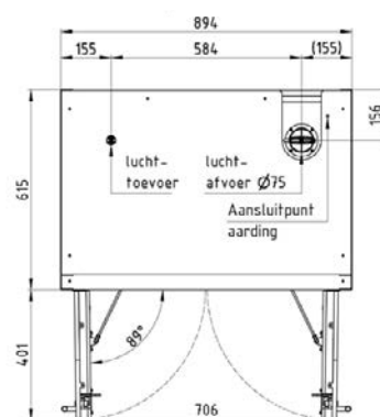
Bovenaanzicht Q90.195.090.CLASSIC
