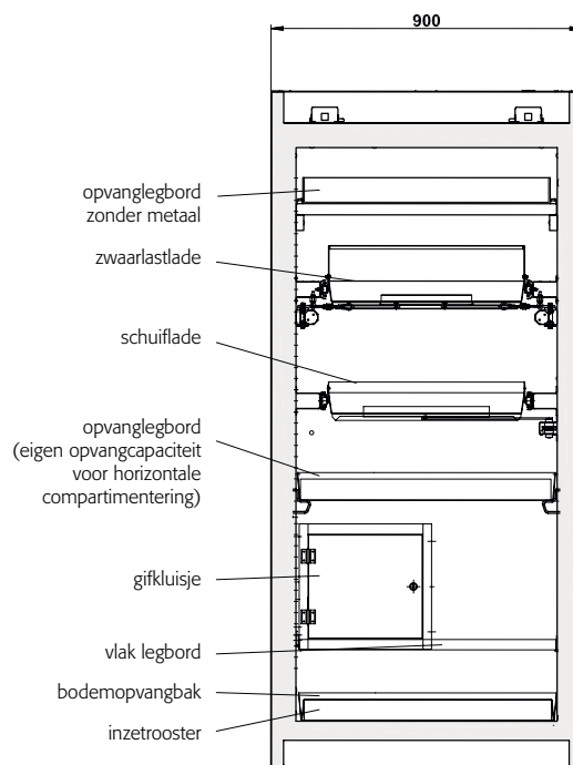
Doorsnede Q90.195.090.CLASSIC
