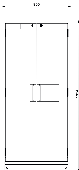
Vooraanzicht Q90.195.090.CLASSIC
