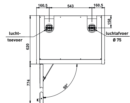
Bovenaanzicht Q30.195.086.CLASSIC
