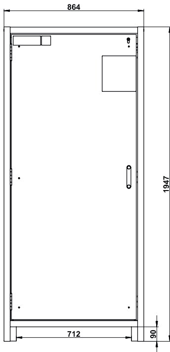
Vooraanzicht Q30.195.086.CLASSIC
