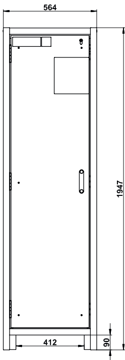
Vooraanzicht Q30.195.056.CLASSIC
