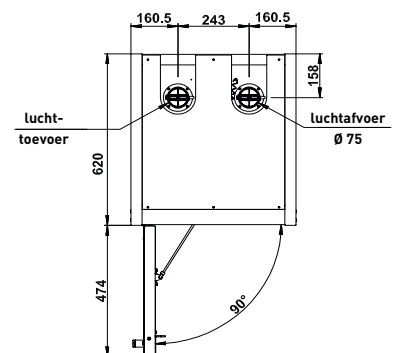
Bovenaanzicht Q30.195.056.CLASSIC
