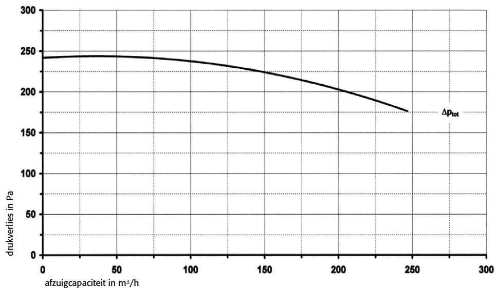
karakteristiek van de ventilatiemodule
