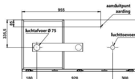
Achteraanzicht K90.060.140.3T
