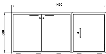
Vooraanzicht K90.060.140.3T
