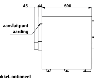
Zijaanzicht K90.060.140.3T
