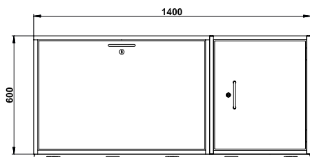
Vooraanzicht K90.060.140.ST
