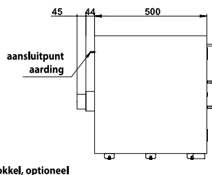
Zijaanzicht K90.060.140.ST
