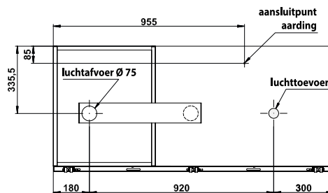
Achteraanzicht K90.060.140.ST
