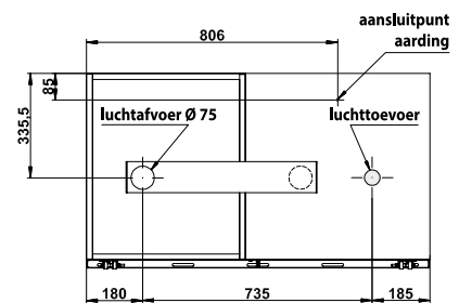
Achteraanzicht K90.060.110.2T
