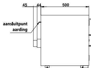
Zijaanzicht K90.060.110.2T
