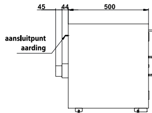
Zijaanzicht K90.060.110.ST
