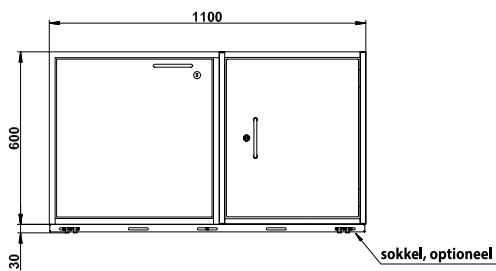
Vooraanzicht K90.060.110.2T
