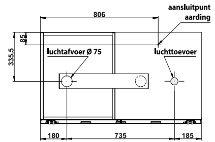
Achteraanzicht K90.060.110.ST
