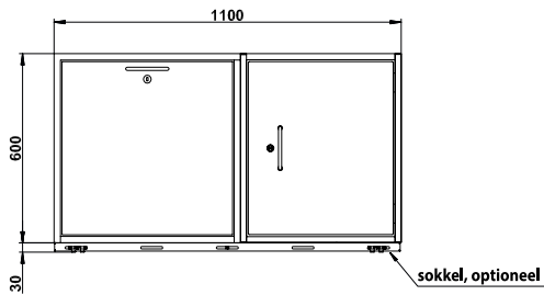
Vooraanzicht K90.060.110.ST
