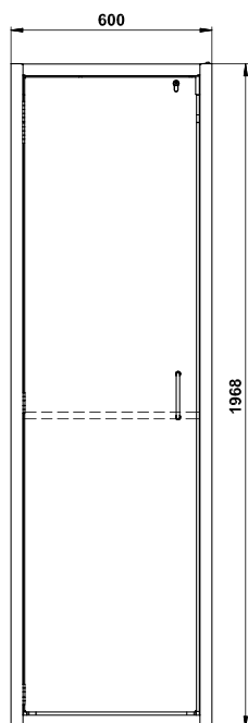
Vooraanzicht K90.196.060.CLASSIC
