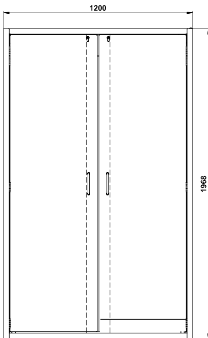
Vooraanzicht K90.196.120.CLASSIC
