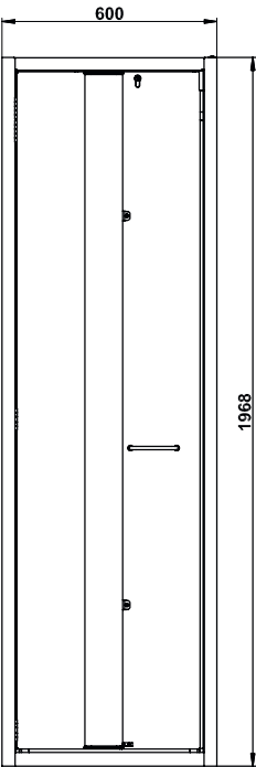
Vooraanzicht S90.196.060.075.PHOENIX Vol. 2
