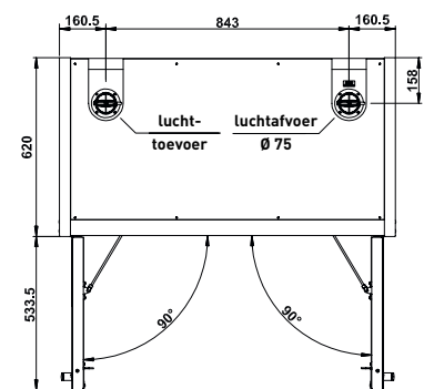
Bovenaanzicht Q30.195.116.CLASSIC
