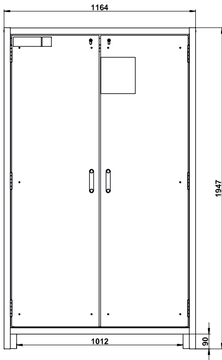
Vooraanzicht Q30.195.116.CLASSIC
