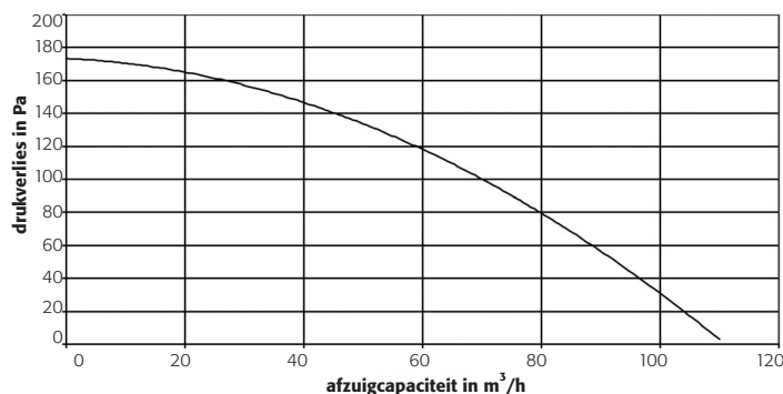
Grafiek ventilatie-opzetunits HF.EA.8677 en HF.EA.11570
