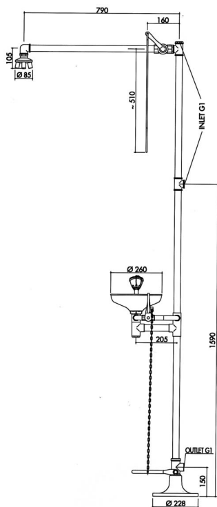
21-1006 + 21-1007 zij-aanzicht
