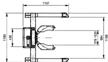
bovenaanzicht
