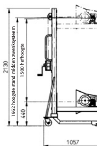
zijaanzicht
