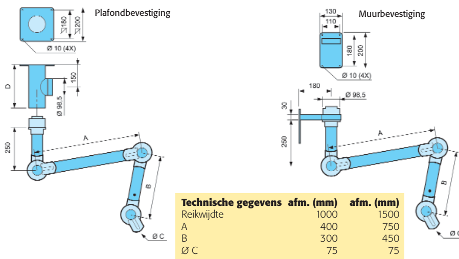
Bronafzuiging voor bevestiging op de muur met muursteun en vlakke kap
